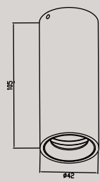
XD2404 8W
