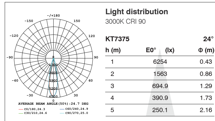
KT7375, 15W, 1476LM
