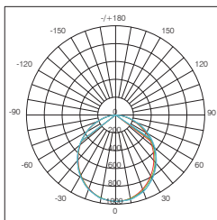
KF1014-35W-3000K-110°
