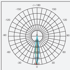
SL367-3W-3000K-10°
