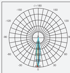
SL367-3W-3000K-10°
