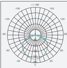
KF1018-16W-3000K-100°
