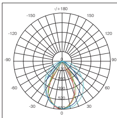
KF1027-37W-3000K-76°
