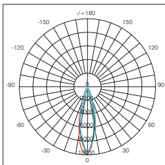
SL362B-28W-3000K-25°
